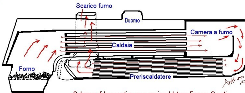
Schema di locomotiva con preriscaldatore Franco-Croști
